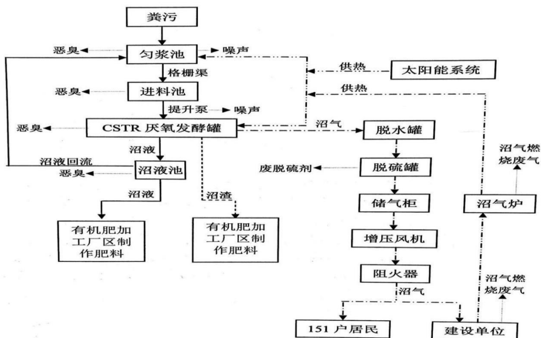
图 2.4 项目工艺流程及产污环节图
